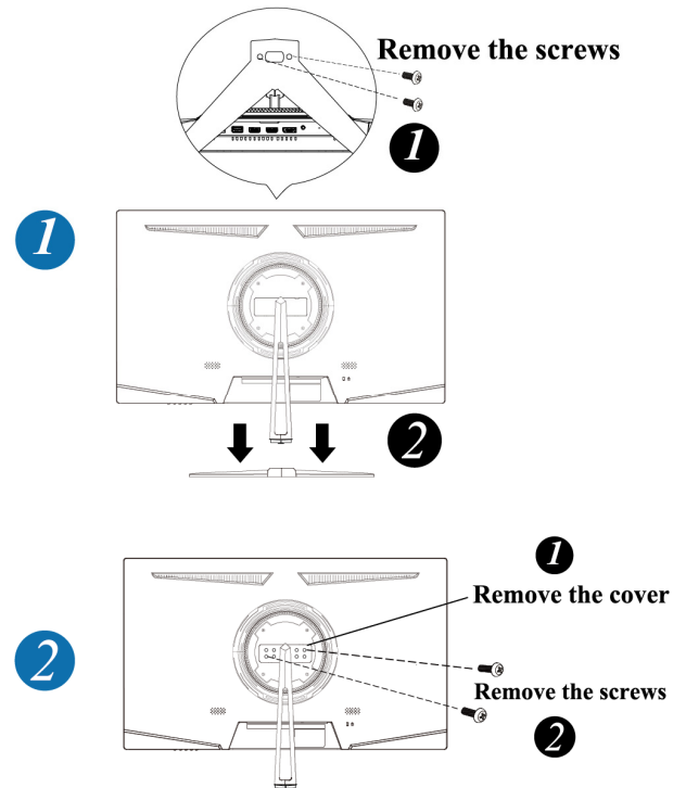
Figure.1. Installer et enlever l'embase
