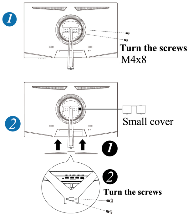
Figure.1. Installer et enlever l'embase
